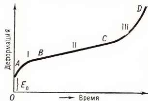
Рис. 1. Пример кривой ползучести.
